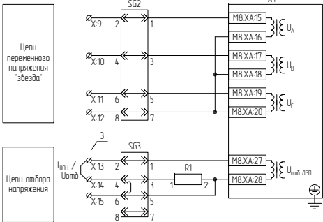
Цепи переменного напряжения
